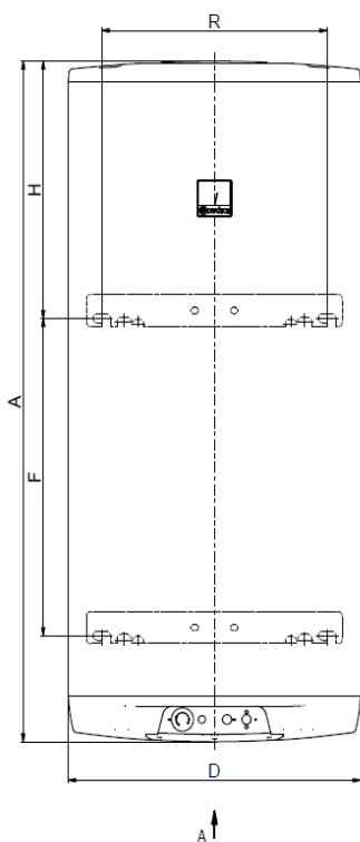
Horný a spodný záves 200 l 4 kotevné skrutky Rozmery 450mm a F pred vŕtaním overiť
