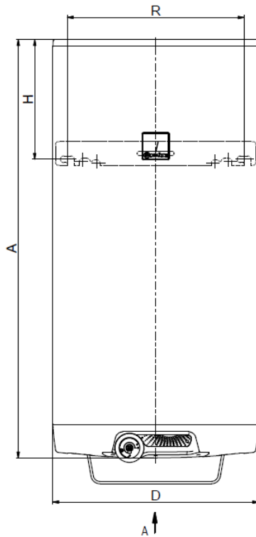
Horný záves 50-160 l 2 kotevné skrutky
