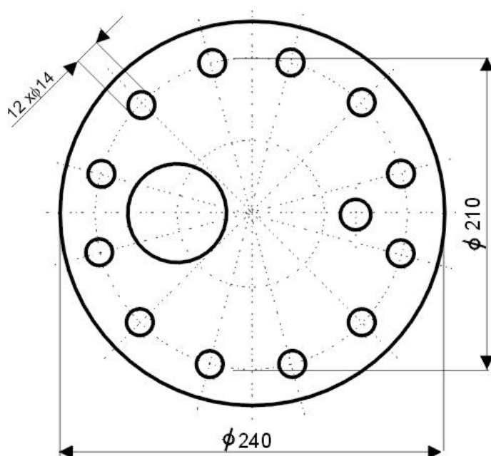
TPK 210 - 12 / 2,2 kW
