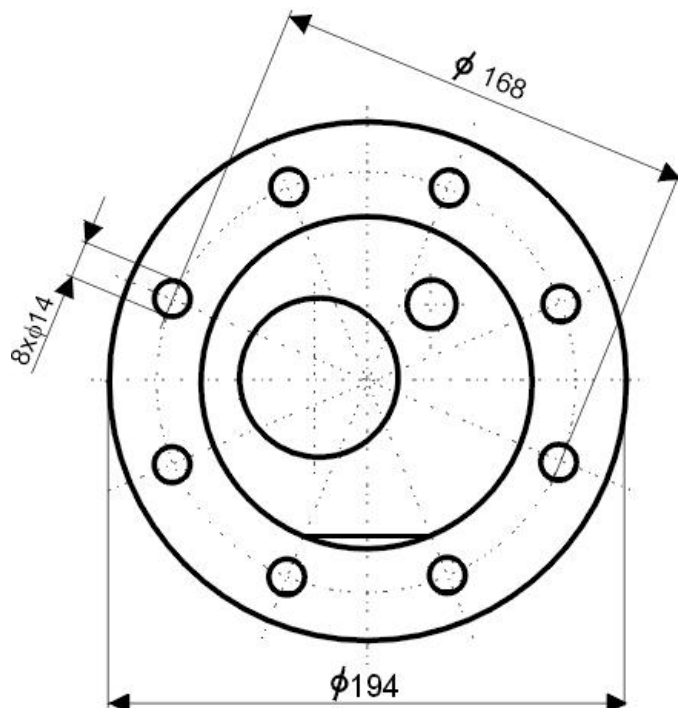
TPK 168 - 8 / 2,2 kW
